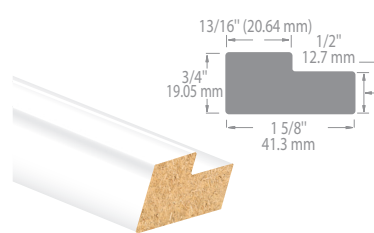
Light Valance 4760
