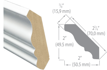
45° Moulding 4123
